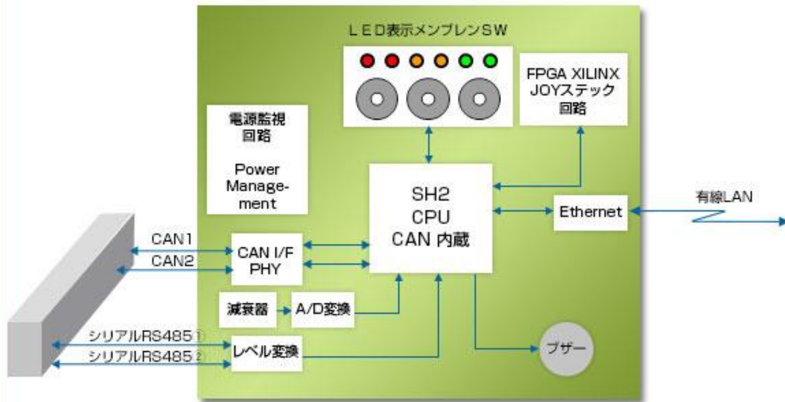
船舶用 AUTO Pilotリモコンブロック図
